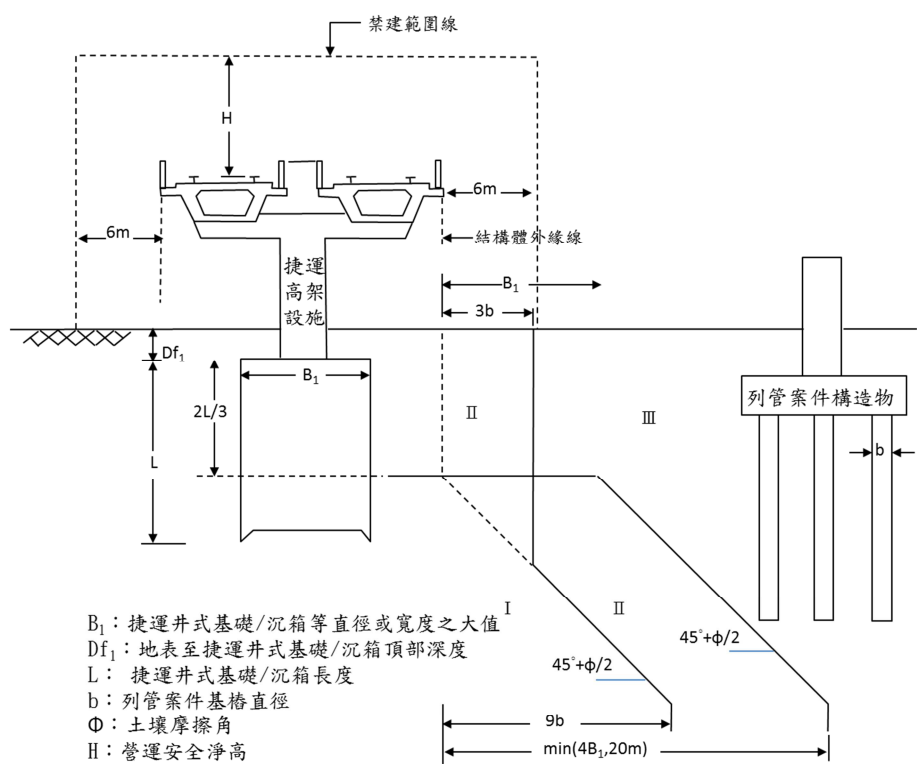
圖三十 列管案件為基樁之分級規範規範圖(高架段適用)
