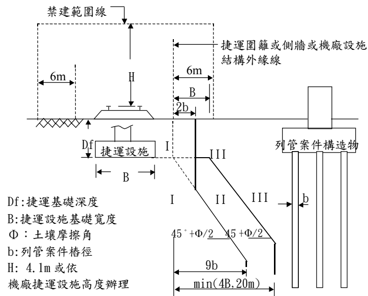
圖十八 列管案件為基樁之分級規範界線圖(地面段、出土段、機廠直接基礎及筏式基礎者適用)
