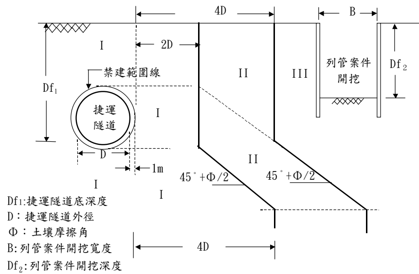
圖一 列管案件為明挖工程之分級規範界線圖(潛盾隧道段適用)
