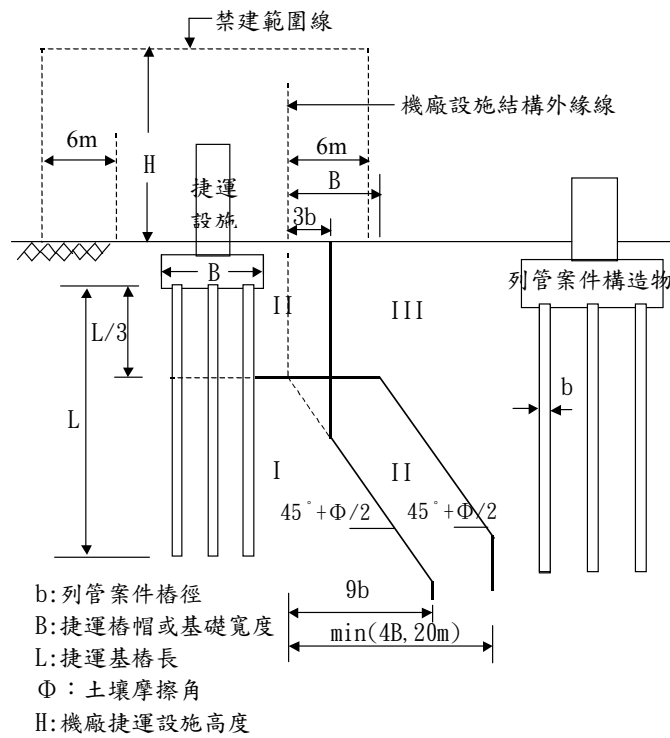
圖二十 列管案件為基樁之分級規範規範圖(機廠樁基結構適用)
