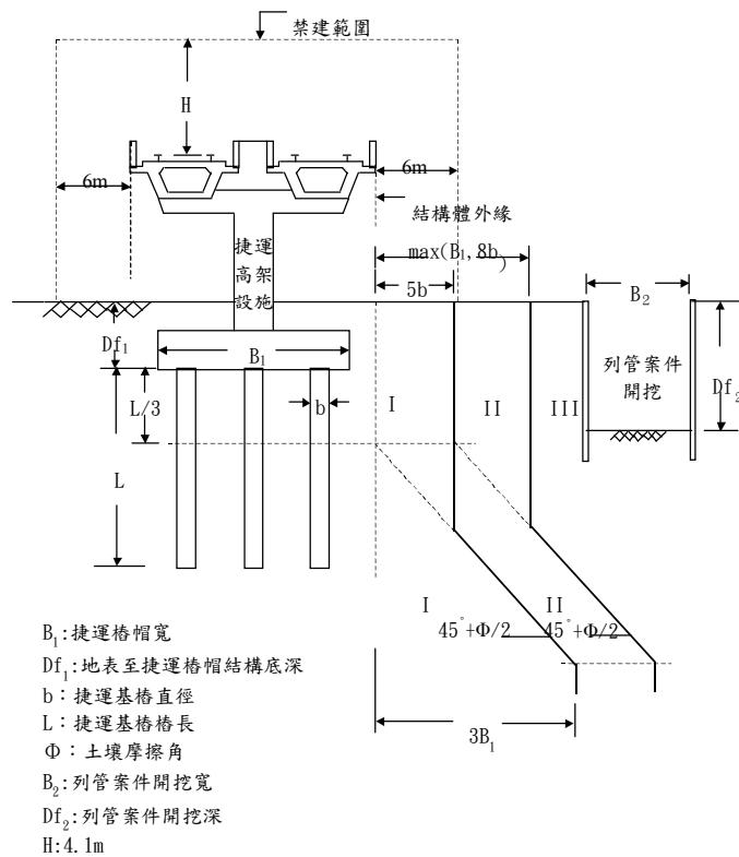
圖四 列管案件為明挖工程之分級規範界線圖(高架段適用)
