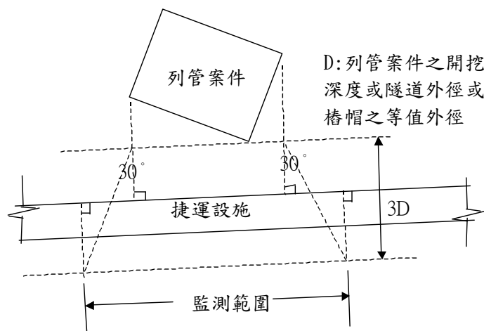
圖 2.1 捷運設施上之監測儀器佈設範圍平面圖 (超出 3D 範圍之捷運設施可不必要裝設)
