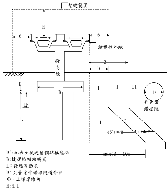
圖九 列管案件為鑽掘隧道之分級規範界線圖(高架段適用)
