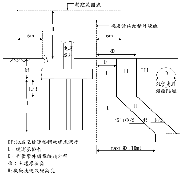
圖九 列管案件為鑽掘隧道之分級規範界線圖(高架段適用)
