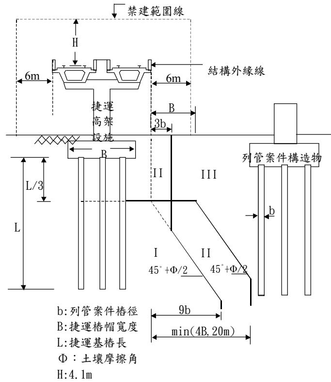
圖十九 列管案件為基樁之分級規範規範圖(高架段適用)
